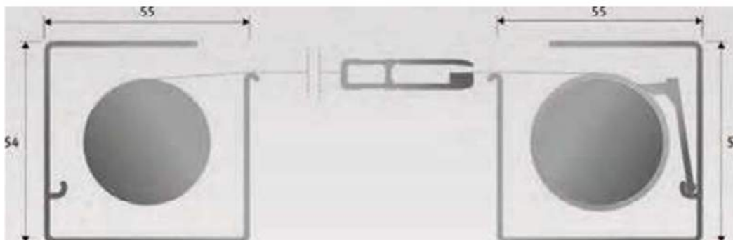
Gegenzug Blende C2 mit Motor
