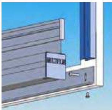
Schraubmontage auf dem Rahmen
