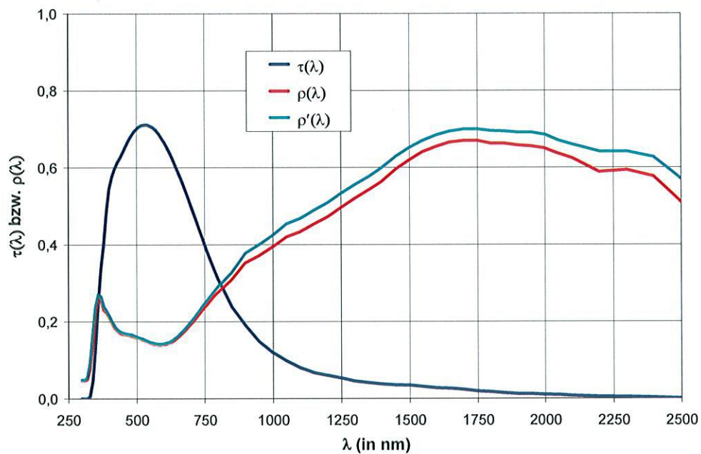
Bild 2: Spektraler Transmissionsgrad \tau(\lambda) bei senkrechtem Lichteinfall und spektraler Reflexionsgrad \rho(\lambda) bei Lichteinfall von außen unter 8^\circ von „eurotherm passiv 42-40 guardian“
