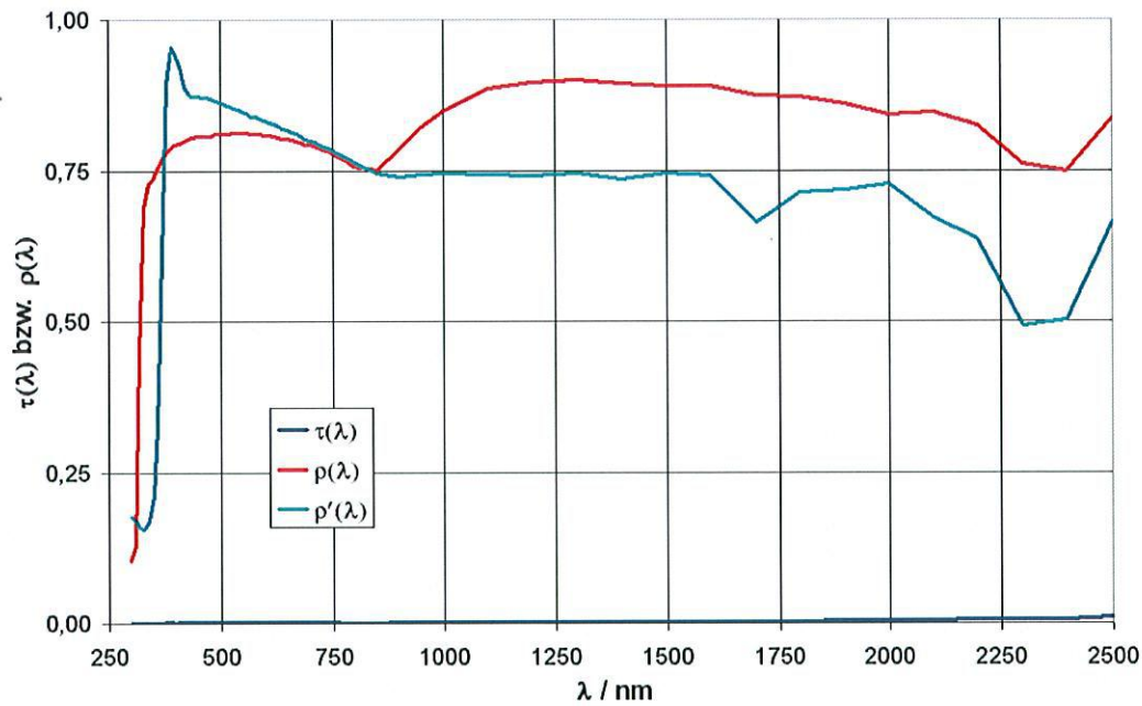
Bild 1: Spektraler Transmissionsgrad \tau(\lambda) bei senkrechtem Lichteinfall und spektraler Reflexionsgrad \rho(\lambda) bei Lichteinfall unter 8^\circ der Folie SiWt002
