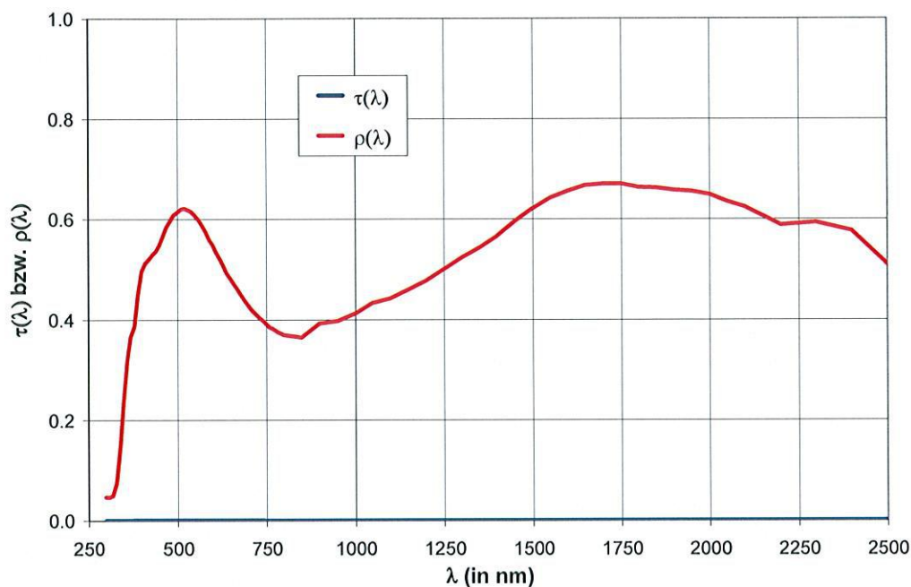
Bild 3: Spektraler Transmissionsgrad \tau(\lambda) bei senkrechtem Lichteinfall und spektraler Reflexionsgrad \rho(\lambda) bei Lichteinfall von außen unter 8^\circ der Kombination „eurotherm passiv 42-40 guardian“ + Folie SiWt002
